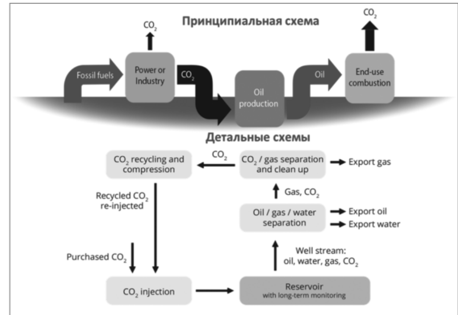
Рис. 6. Схемы \text{CO}_2 -процессов повышения нефтеотдачи пласта
