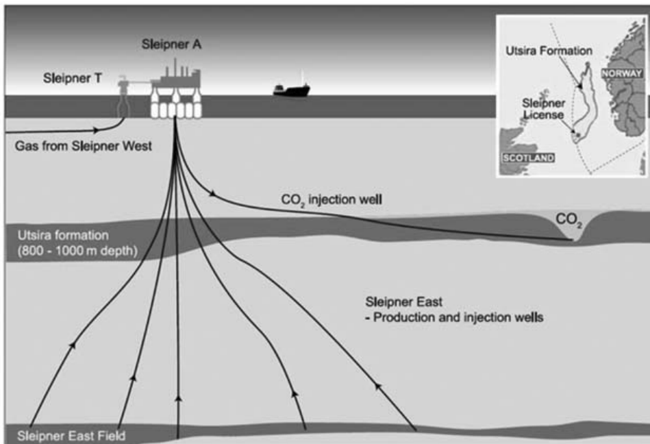
Рис. 5. Схема подземного хранилища двуокиси углерода в выработанном месторождении Слейпнер, Северное море
